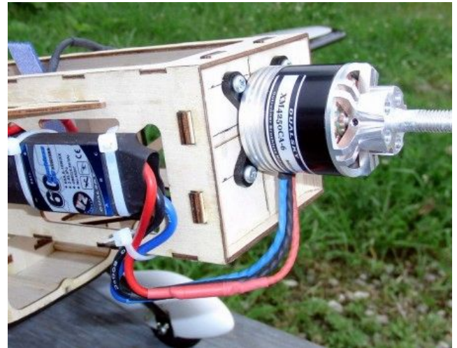
防火壁を移動させてちょうどいい長さにネジを締めて固定します
